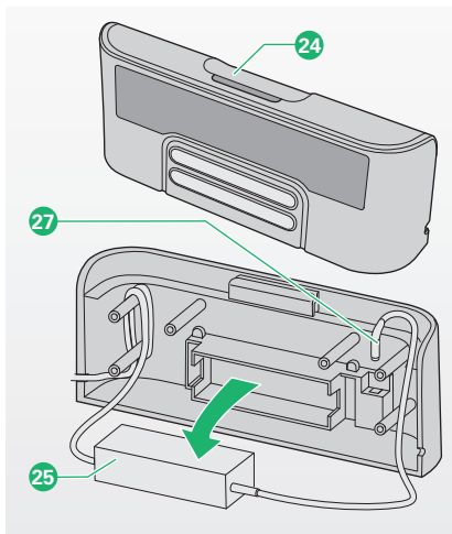
Obrázek 2.7 Vyjmutí síťového zdroje ze základny
